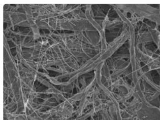
SEM 100x
